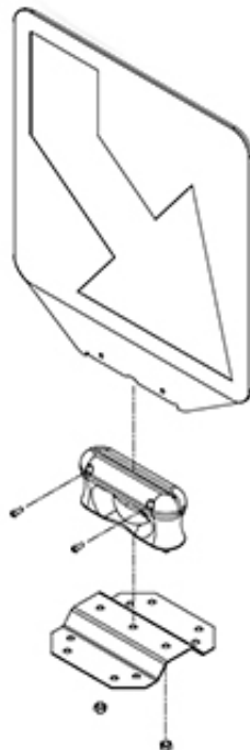
Platine de fixation: Chevilles et tirefonds fournis
